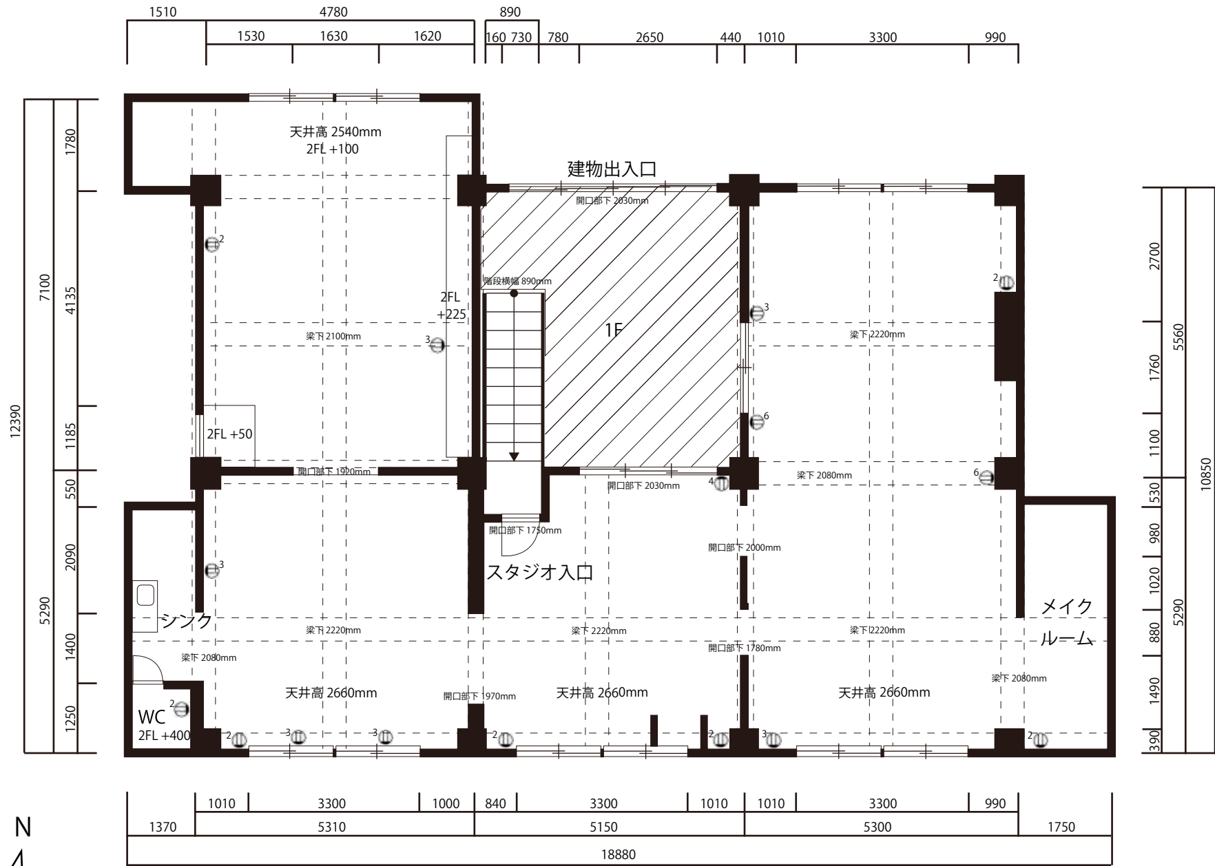
旧海岸 第16スタジオ (2F) 平面図 1/100
